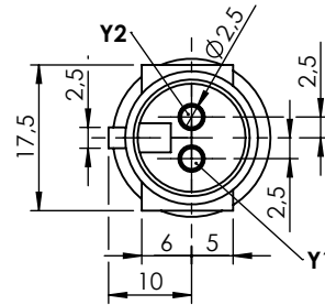
VIEW / VISTA Y SCALE / ESCALA 1 : 1
