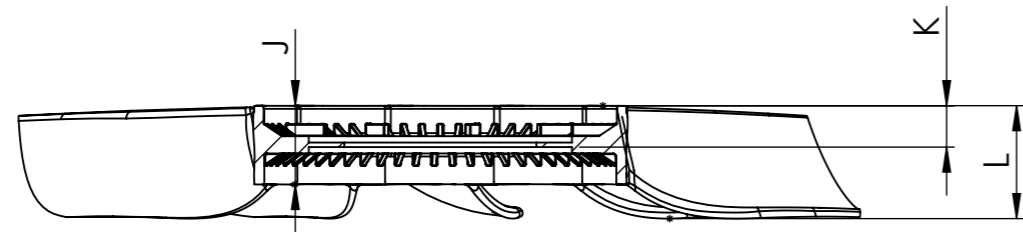
SECCIÓN A-A ESCALA 1 : 5
