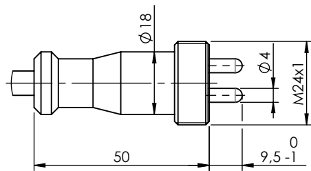
DETAIL / DETALLE Y SCALE / ESCALA 2 : 3
