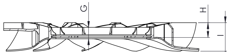
SECCIÓN A-A
