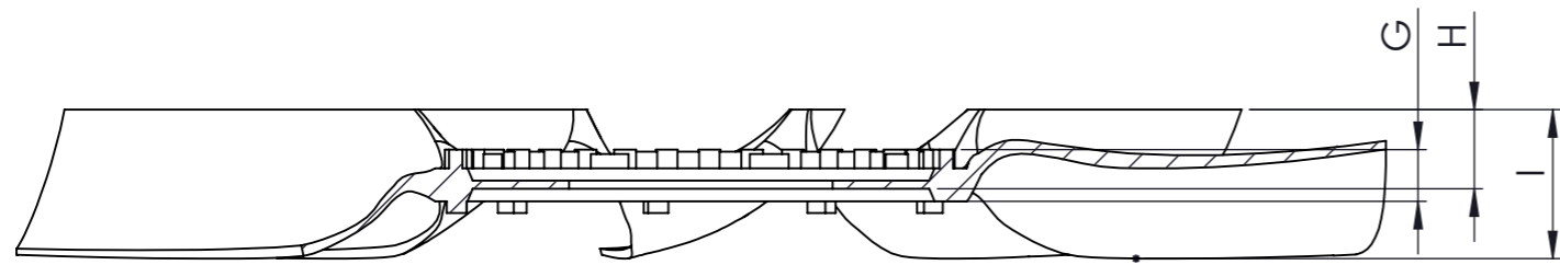
SECTION A-A
