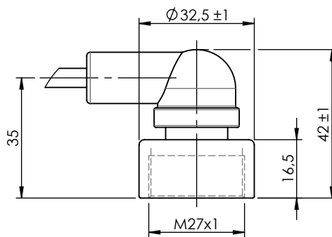
DETAIL / DETALLE Y SCALE / ESCALA 2 : 3
