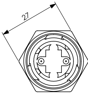
VISTA A
