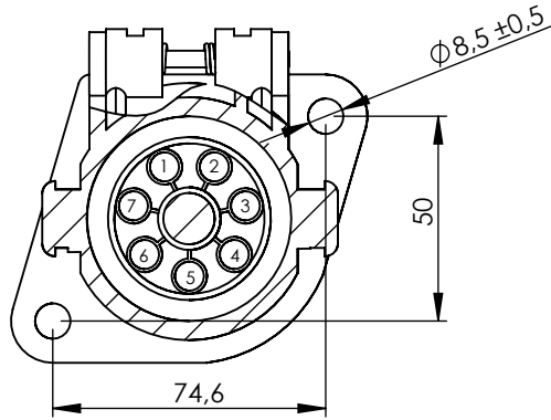
VIEW/VISTA B ESCALA 1 : 2
