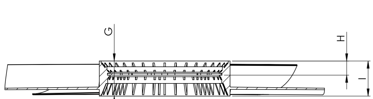
SECCIÓN A-A ESCALA 1:5
