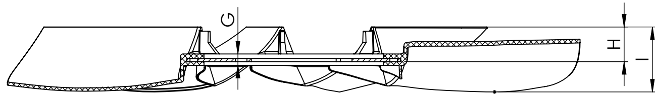
SECTION A-A
