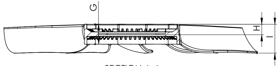
SECTION A-A
