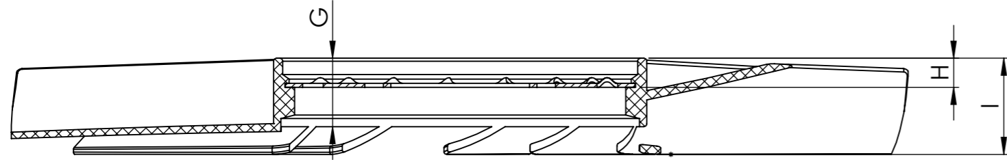
SECTION A-A
