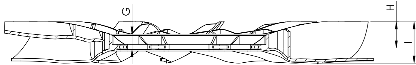
SECCIÓN A-A
