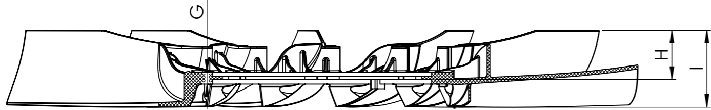
SECTION A-A
